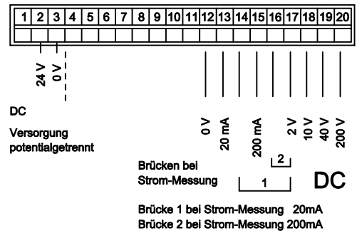
Steckbare Schraubklemmenleiste
